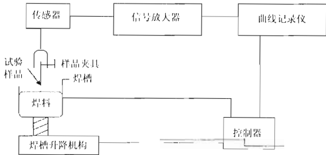
图 208-1 框图
